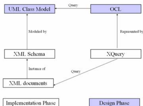
Fig1: UML/OCL, XML/XQuery mapping framework
